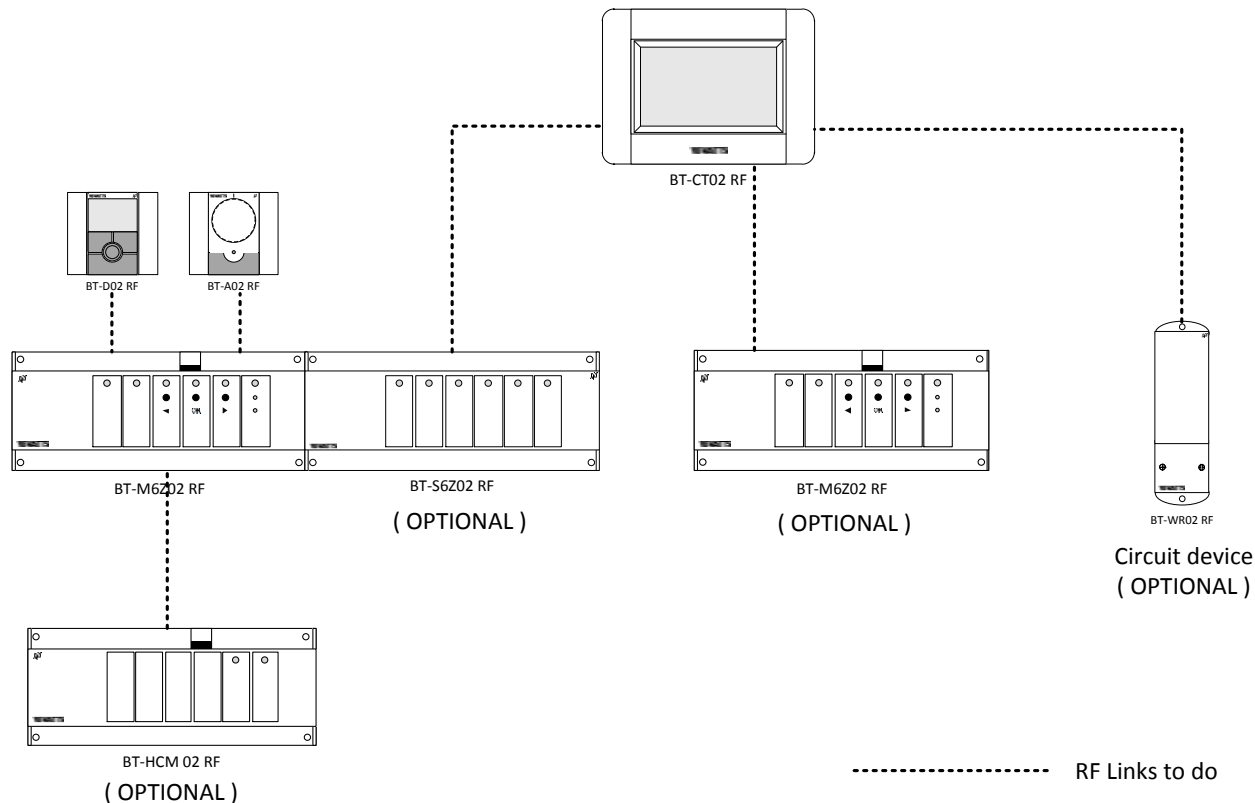
Esempio di "impianto centralizzato"
